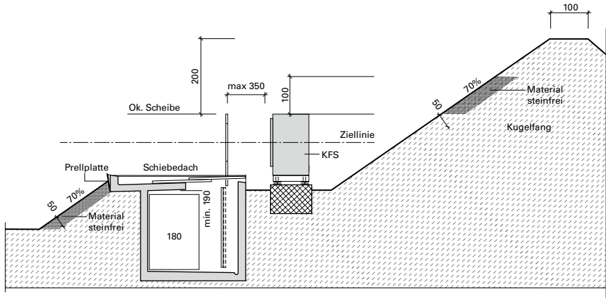
Abb. 42: Aufgeschütteter Kugelfang
