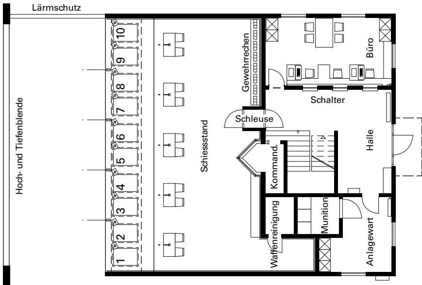
Abb. 16: Schützenhausgrundriss
