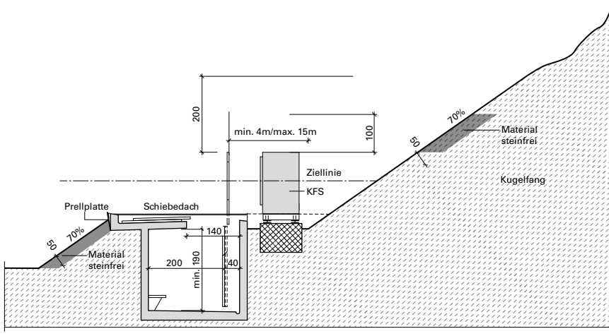
Abb. 41: Natürlicher Kugelfang
